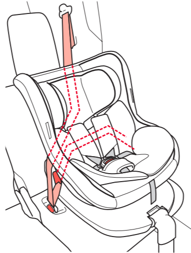
〈後席左側の取り付けイメージ〉
